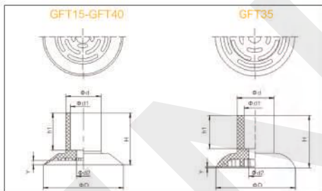
外螺纹安装方式 M
